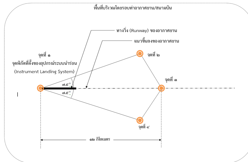
รูปที่ ๑ พื้นที่ปลอดภัยการรบกวนการใช้คลื่นความถี่สำหรับลระดับเพดานบินและร่อนลงจอดของอากาศยาน
